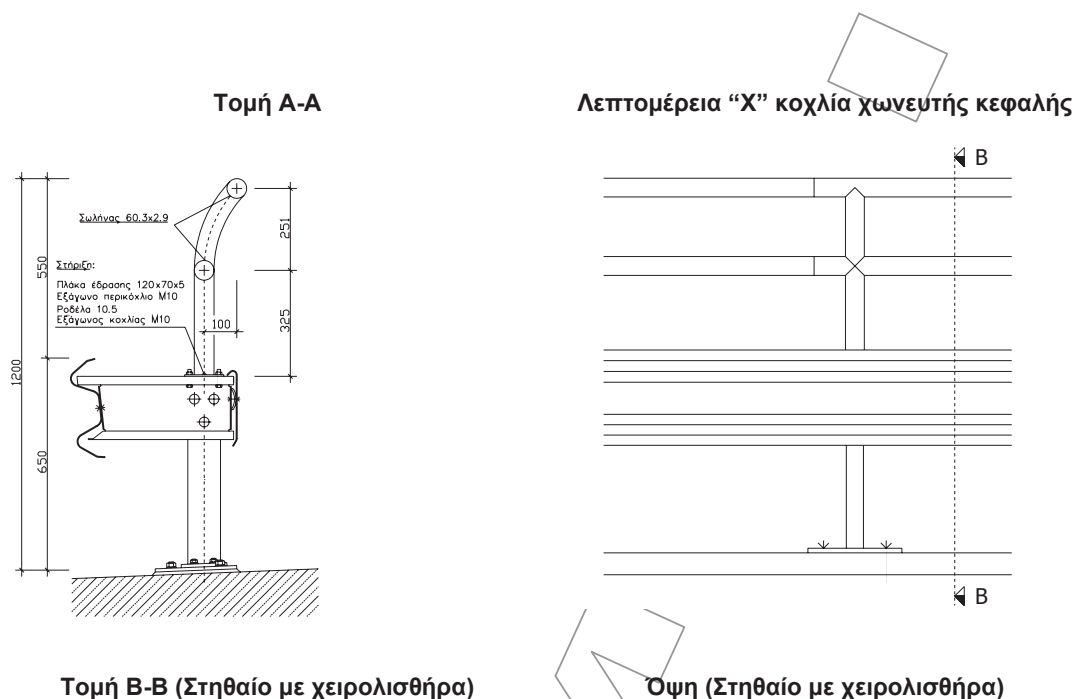
Σχήμα 1 – Ενδεικτική διάταξη στήριξης ορθοστατών μεταλλικών στηθαίων ασφαλείας
