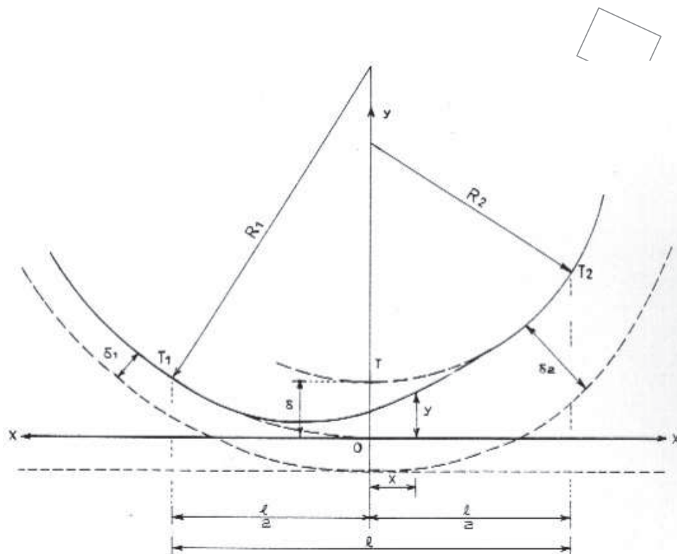
Σχήμα 4 – Παραβολική συναρμογή μεταξύ δύο συνεχόμενων κυκλικών καμπυλών
