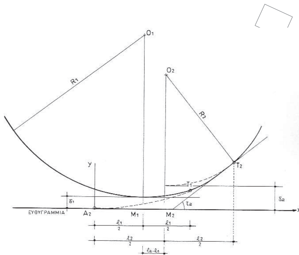
Σχήμα 5 – Παραβολική συναρμογή μεταξύ δύο ομόστροφων κυκλικών καμπυλών ακτίνας R_1 & R_2 ( R_1 > R_2 ) με μικρή ενδιάμεση ευθυγραμμία
