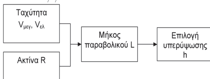
Σχήμα 1 – Διαδικασία σχεδιασμού καμπυλών
