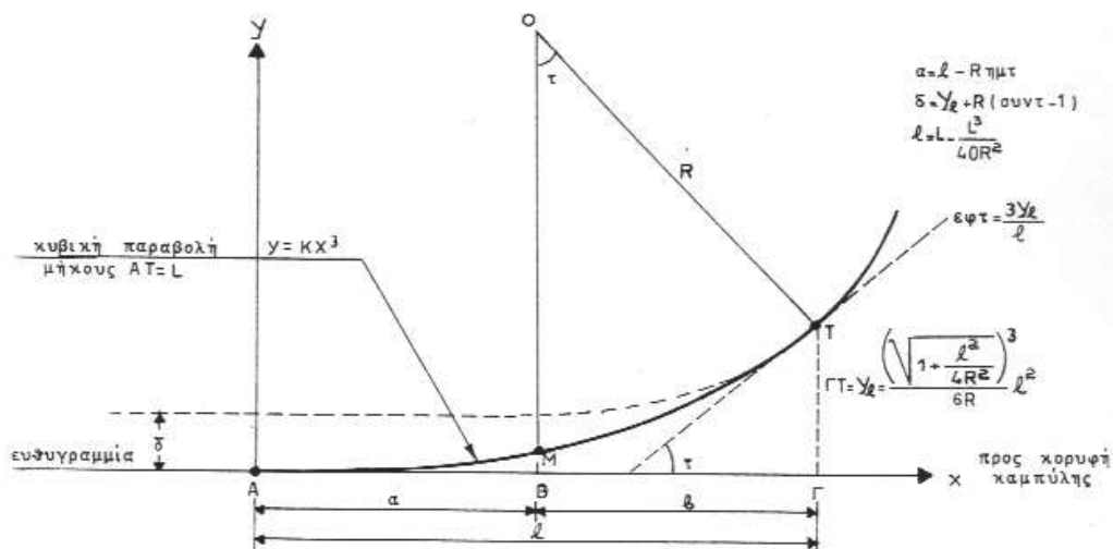
Σχήμα 3 – Παραβολική συναρμογή μεταξύ ευθυγραμμίας και κυκλικής καμπύλης
