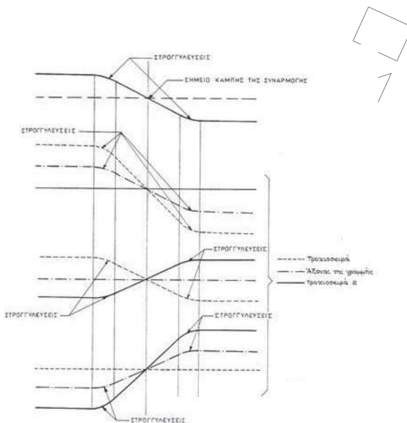
Σχήμα 10 – Μηκοτομή τροχιοσειρών
