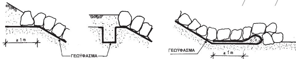
Σχήμα 1 – Ενδεικτικές διατάξεις αγκύρωσης γεωϋφάσματος
