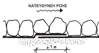
Σχήμα 2 - Επικάλυψη γεωϋφάσματος
