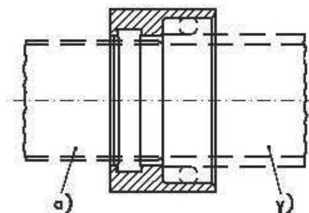
Σχήμα 9 – Μεταβατικός σύνδεσμος
