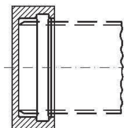
Σχήμα 12 – Τμήμα φραγής
