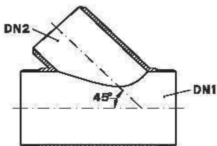
Σχήμα 4 – Διακλάδωση 45°
