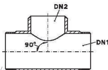
Σχήμα 5 – Διακλάδωση 90°
