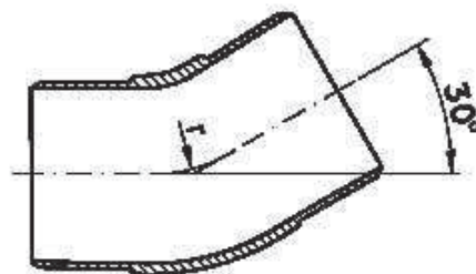
Σχήμα 7 – Καμπύλη 30°
