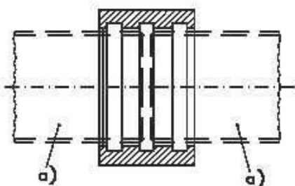
Σχήμα 2 – Τυπικός σύνδεσμος
