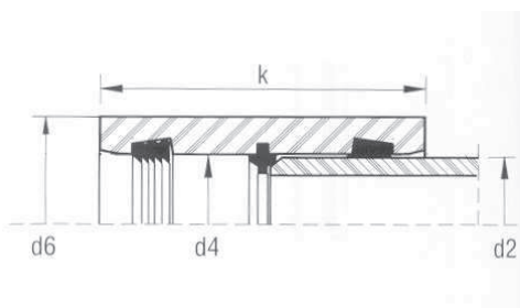
Σχήμα 1 – Σύνδεσμος REKA
