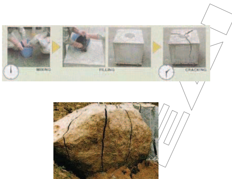
Σχήμα 1 - Διάσπαση υλικών με διογκούμενα υλικά (αθόρυβα εκρηκτικά)
