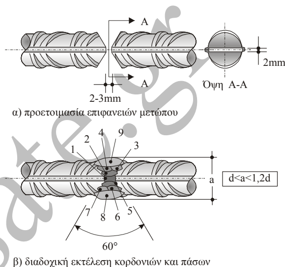
Σχήμα 8-2 Μετωπική σύνδεση με συγκόλληση τόξου (λοξοτομή διπλού-V στις δύο ράβδους σε οριζόντια θέση)
