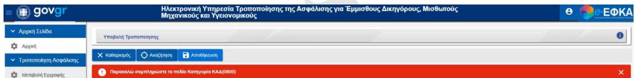
Εικόνα 1 Μήνυμα Σφάλματος 1
