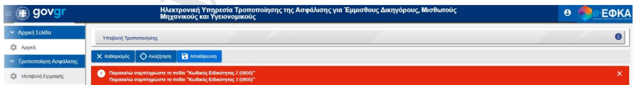
Εικόνα 2 Μήνυμα Σφάλματος 2
