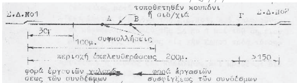
Σχήμα 14 - Θέση συγκολλήσεως γ
