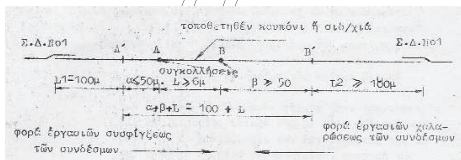
Σχήμα 13 - Θέση συγκολλήσεως β
