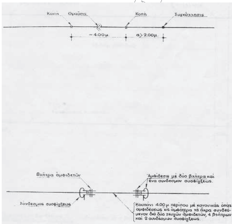
Σχήμα 1 - Προσωρινή αποκατάσταση θραύσης τύπου «Α»
