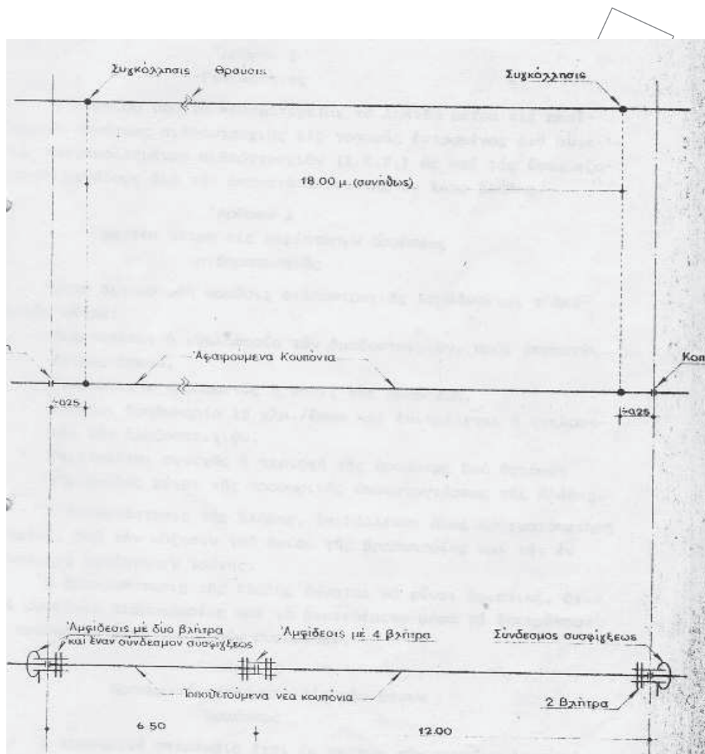
Σχήμα 2 - Προσωρινή αποκατάσταση θραύσης τύπου "B"
