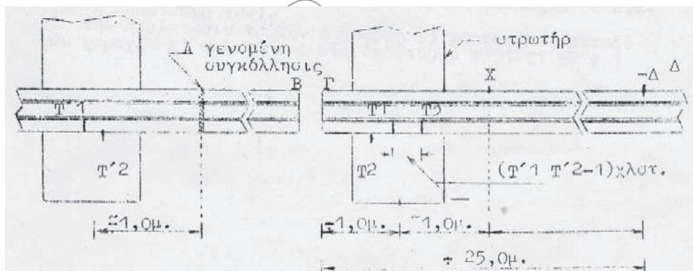
Σχήμα 11 - Μετακίνηση των χαραγών Τ1' και Τ1, στο πέλας της σιδηροτροχιάς που είναι στη γραμμή, λόγω συστολής της ράβδου 12
