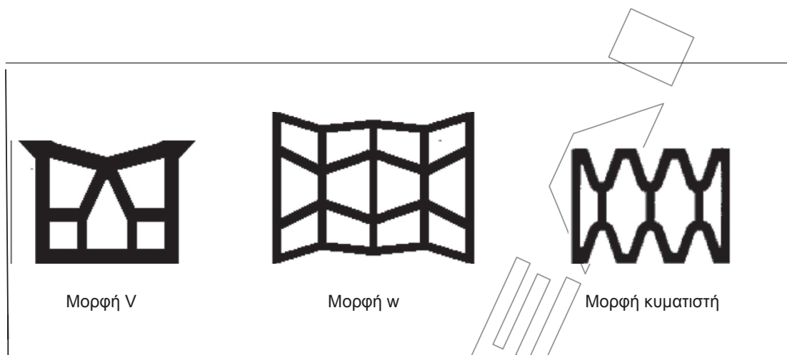
Σχήμα 1 – Προδιαμορφωμένα υλικά πλήρωσης αρμών κυψελωτής δομής
