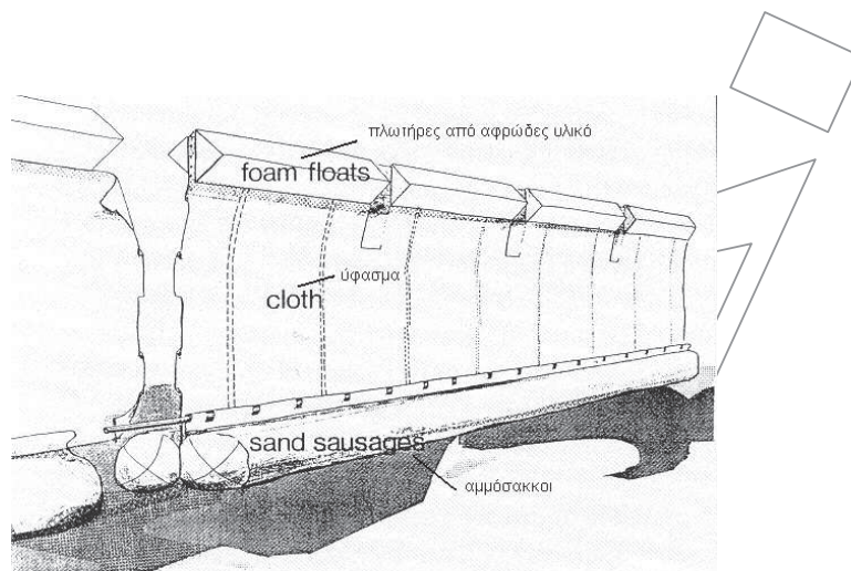
Σχήμα 2: Τυπική διάταξη πλωτού διαφράγματος
