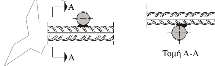
Σχήμα 8 - Σύνδεση σταυρωτά
