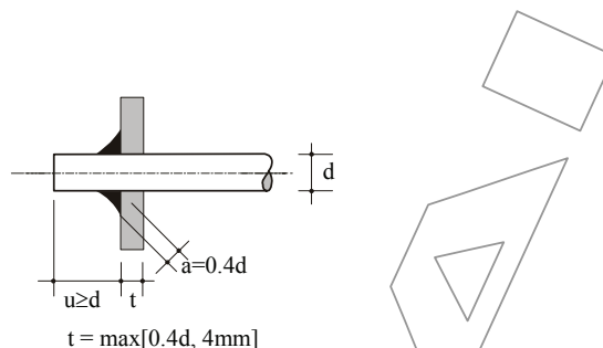
Σχήμα 12 - Ράβδος περαστή στο έλασμα
