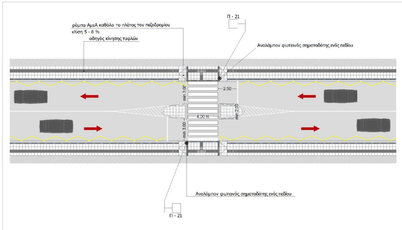
Σχήμα 5: Ενδεικτική τοπική κεντρική νησίδα ως καταφύγιο πεζών.
