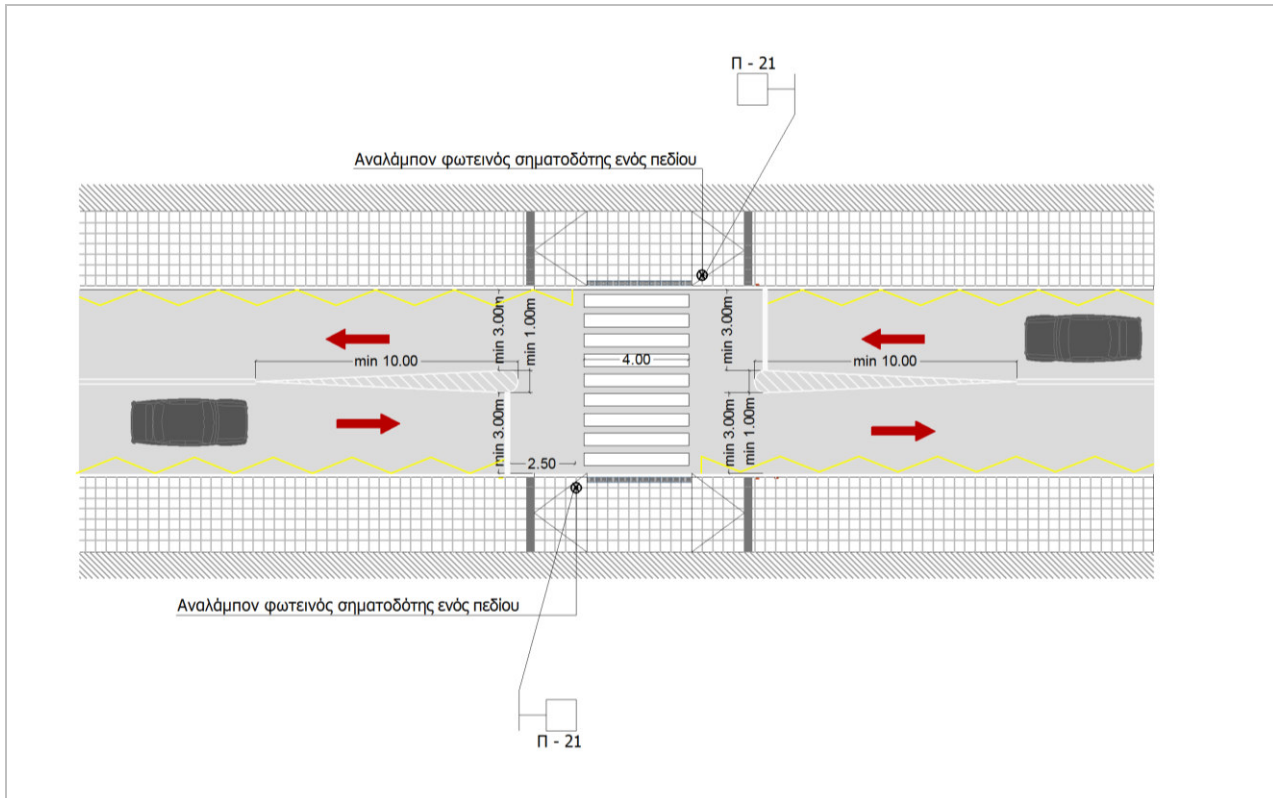
Σχήμα 6: Ενδεικτική στένωση οδοστρώματος με διαγράμμιση
