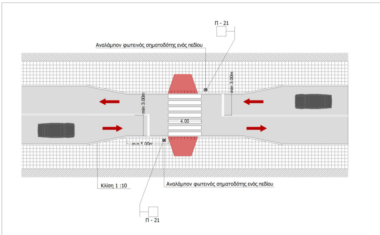
Σχήμα 7: Ενδεικτική στένωση οδοστρώματος με προεξοχή στο οδόστρωμα.
