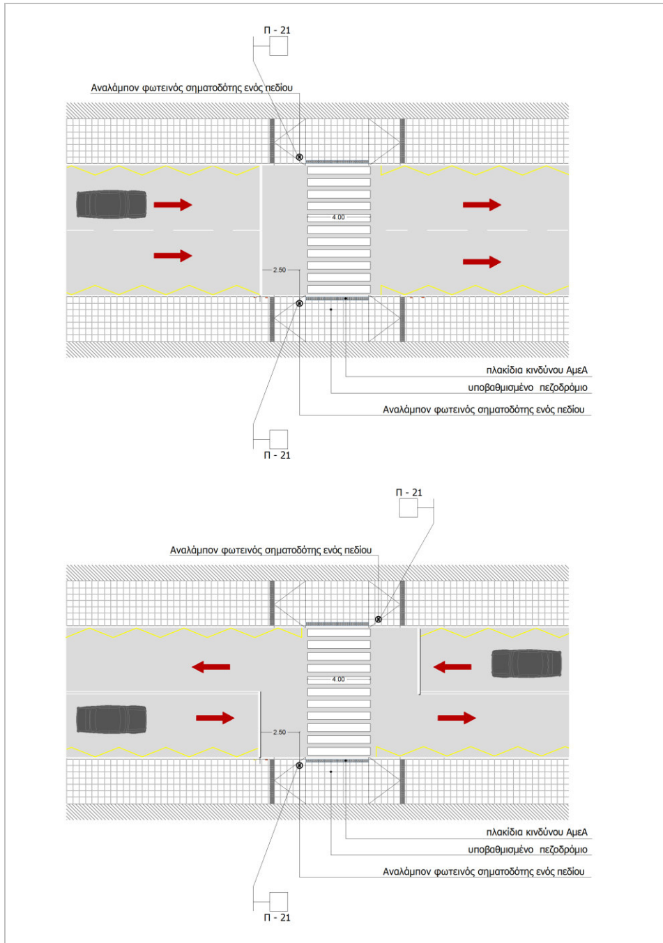
Σχήμα 4: Τυπική διαμόρφωση πεζοδιάβασης με χρήση αναλάμποντος σηματοδότη
