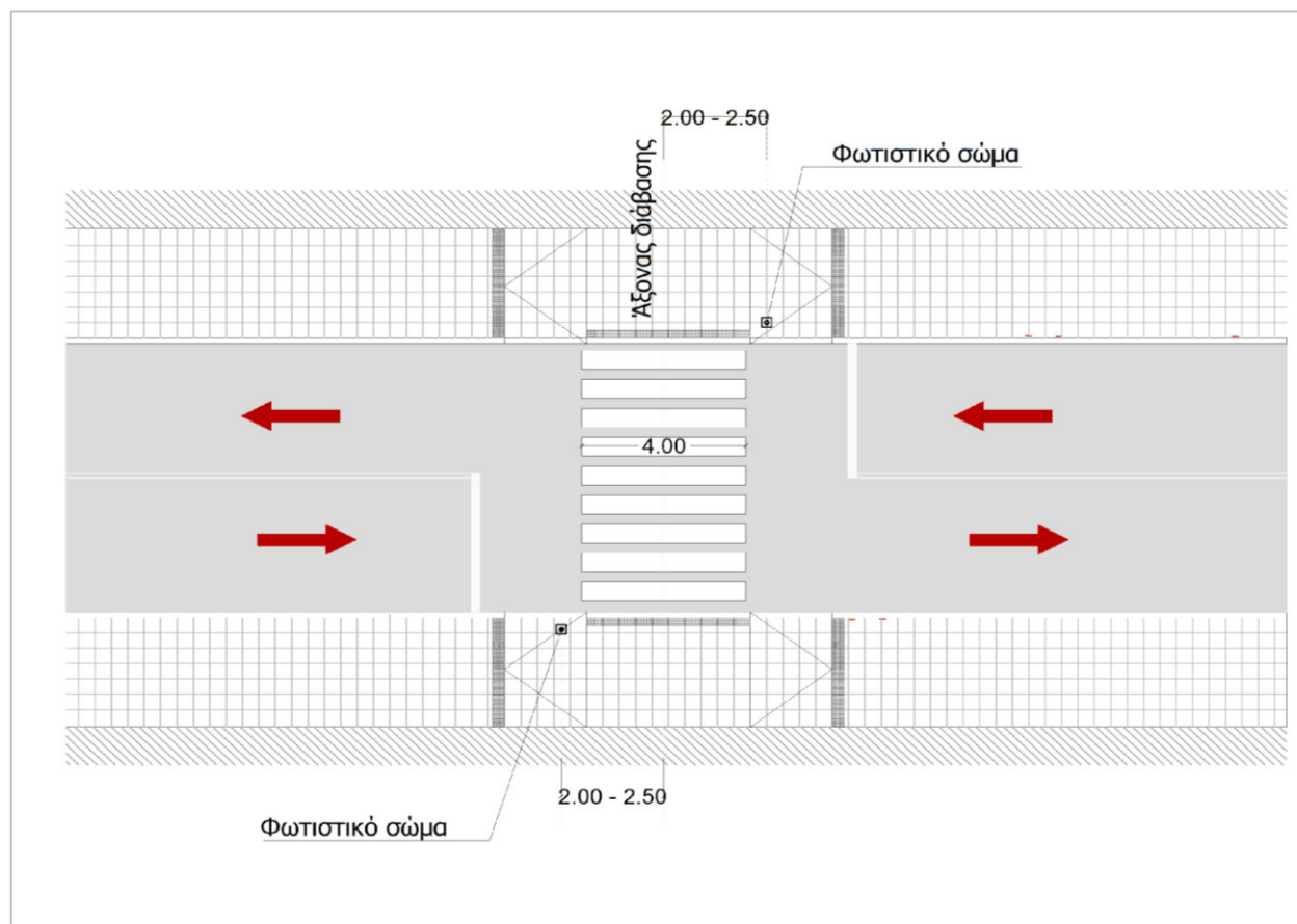
Σχήμα 10: Διάβαση πεζών σε οδό διπλής κυκλοφορίας
