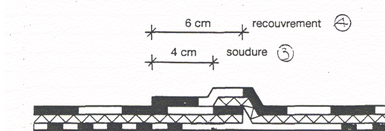
Σχήμα 9 - Κόλληση μεταξύ των φύλλων των ρολλών: στην ζώνη επικάλυψης των φύλλων δεν θα πρέπει να κολλείται η μεμβράνη στο υπόστρωμά της.
