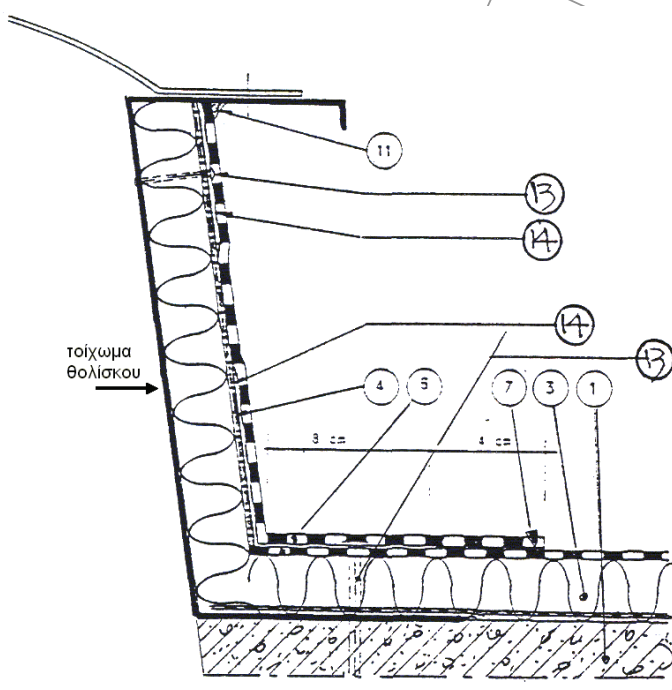
Διάταξη κατάληξης μεμβράνης σε θερμομονούμενα τοιχώματα θόλου που εδράζεται επί της πλάκας.
