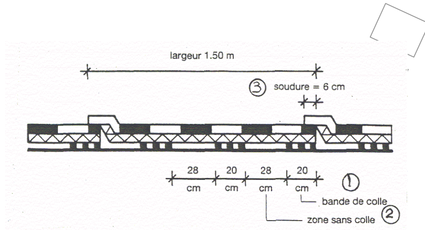
Σχήμα 7 - Κόλληση των μεμβρανών στο κεντρικό τμήμα δώματος-στέγης: λωρίδες κόλλησης 20 cm- λωρίδες χωρίς κόλληση 28 cm, πλάτος ζώνης 1,50 m.
