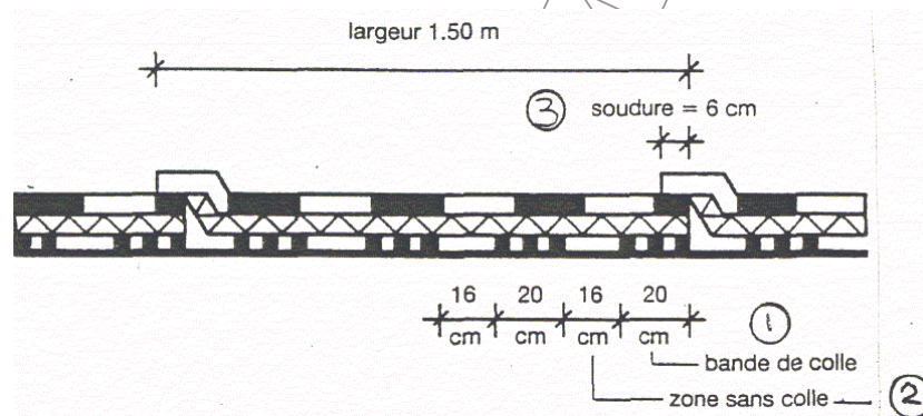
Σχήμα 8 - Κόλληση των μεμβρανών στην περιμετρική ζώνη δώματος-στέγης: πλάτος ζώνης 1,50, όπου εφαρμόζεται παρόμοια κόλληση όταν το πλάτος της κατασκευής είναι \leq 15 m. Στην αντίθετη περίπτωση είναι 3 m. Λωρίδα κόλλησης 20 cm. Λωρίδα χωρίς κόλληση 16 cm.
