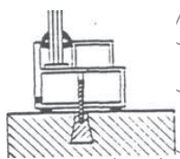
Σχήμα 11 - Πατούρα υαλοστασίου αλουμινίου με ή χωρίς διάταξη διακοπής θερμικών γεφυρών, στερεούμενου (έστω και κατά το ένα άκρο) απ' ευθείας σε τοίχο ή σε πατούρα σκυροδέματος
