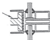
Σχήμα 14 - Πατούρα σταθερού υαλοστασίου αλουμινίου ή χάλυβος λεπτών διατομών με ή χωρίς
