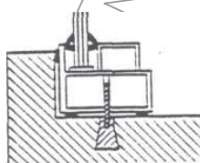
Σχήμα 12 - Πατούρα υαλοστασίου αλουμινίου με ή χωρίς διάταξη διακοπής θερμικών γεφυρών, στερεούμενου (έστω και κατά το ένα άκρο) απ' ευθείας σε ένα τοίχο ή σε σχηματιζόμενη γωνία από τοίχο ή σε πατούρα σκυροδέματος
