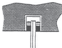
Σχήμα 15 - C 1 Πατούρα διαμορφωμένη σε ανόργανα υλικά (σκυρόδεμα, σπτοπλινθοδομή, λιθοδομή)
